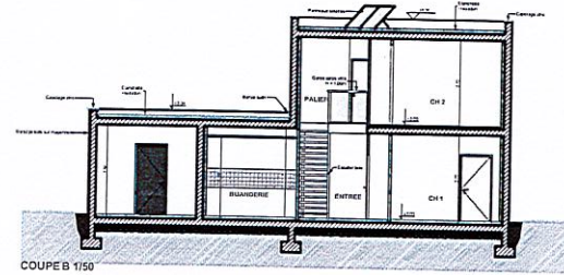
COUPE B 1/50
