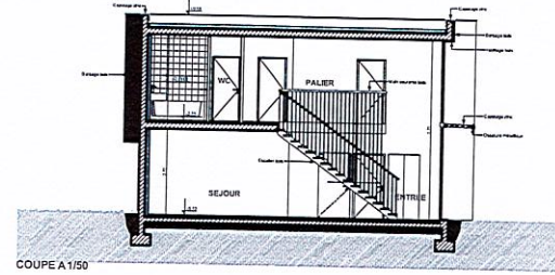
COUPE A 1/50
