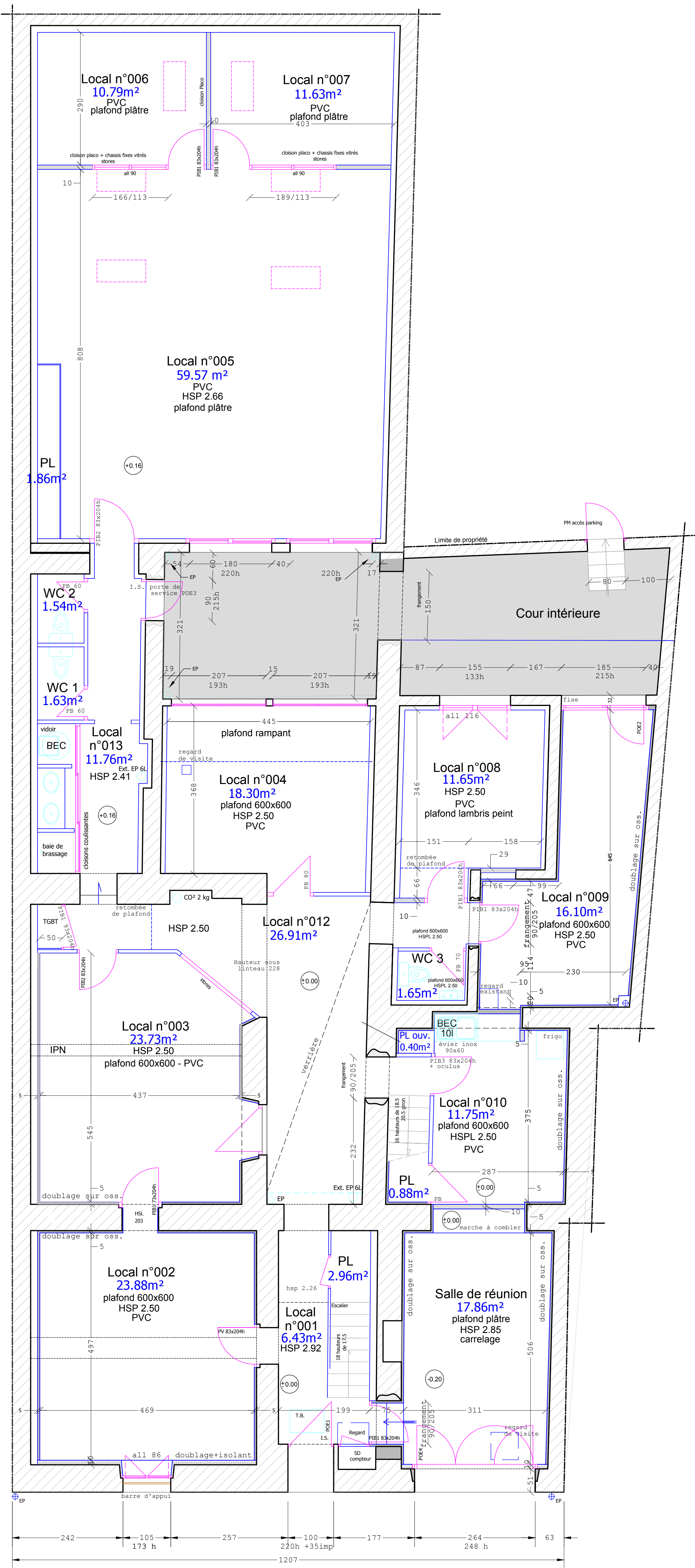
RDC
