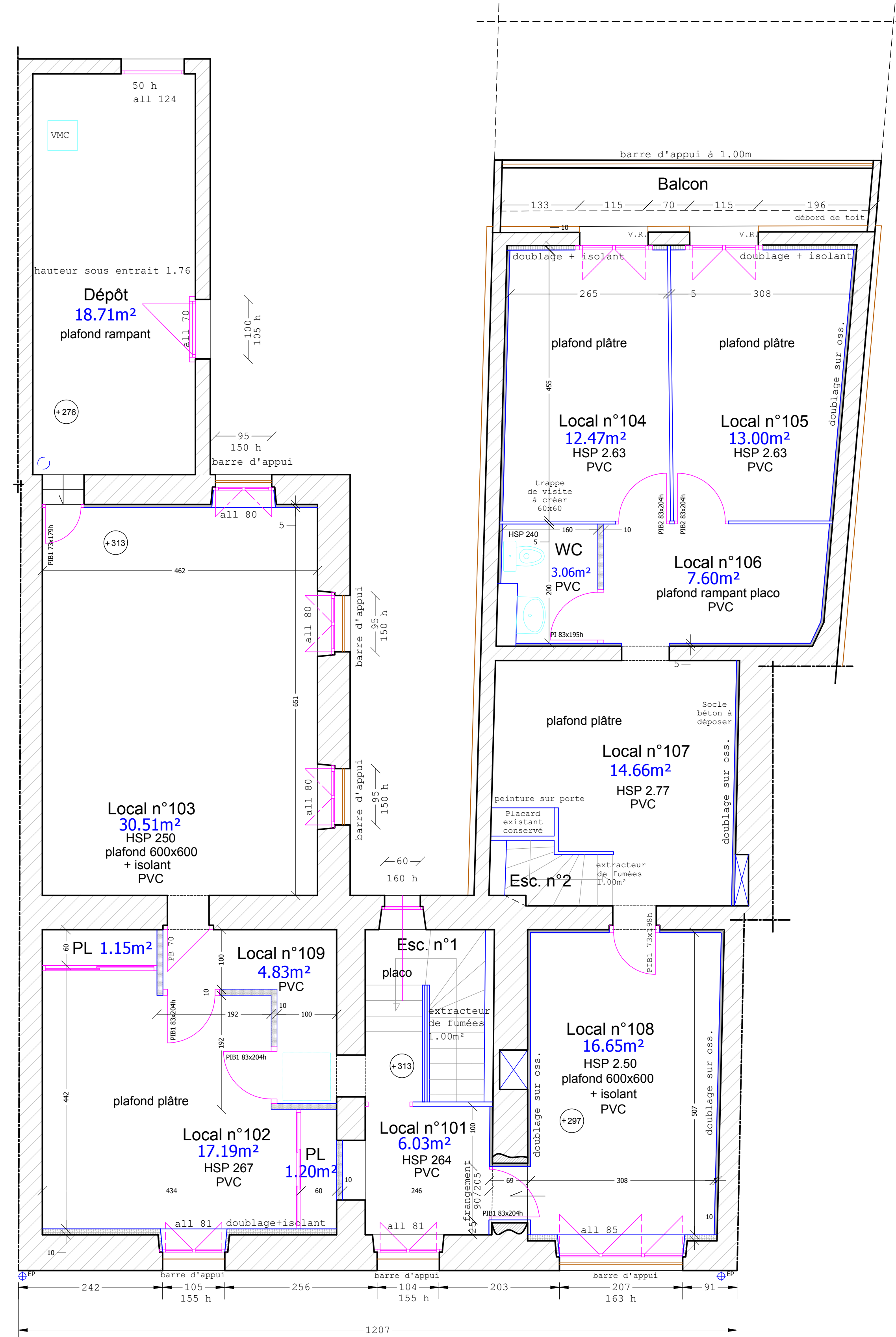
Etage
